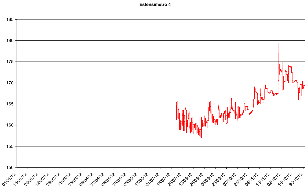
Figura n.8- Spostamento dell'estensimetro 4.
