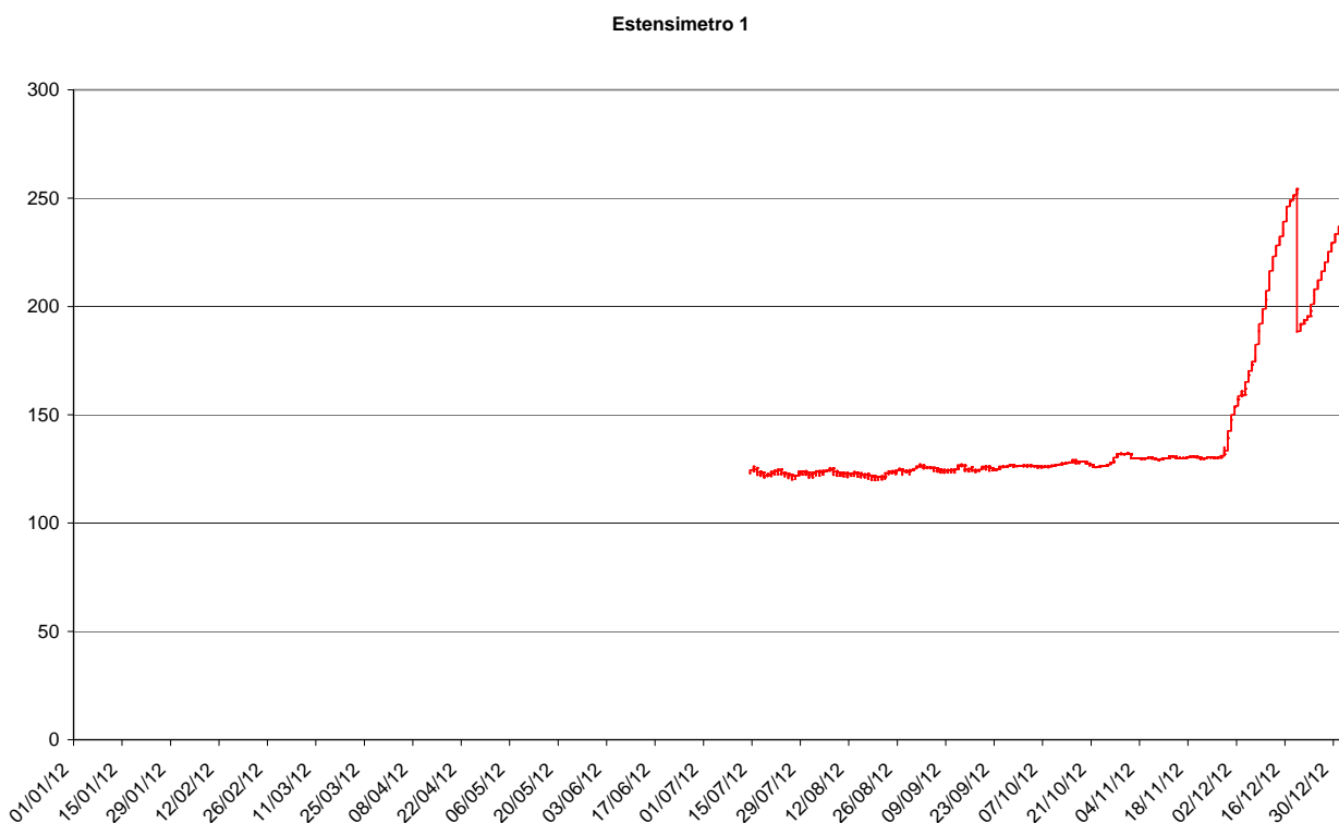
Figura n. 5- Spostamento dell'estensimetro 1.
