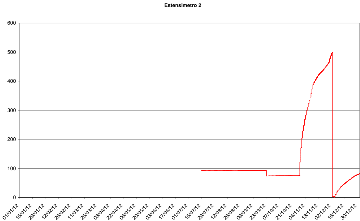
Figura n.6- Spostamento dell'estensimetro 2.
