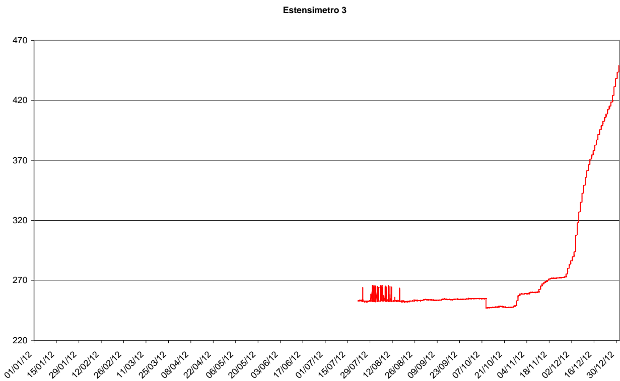
Figura n.7- Spostamento dell'estensimetro 3.
