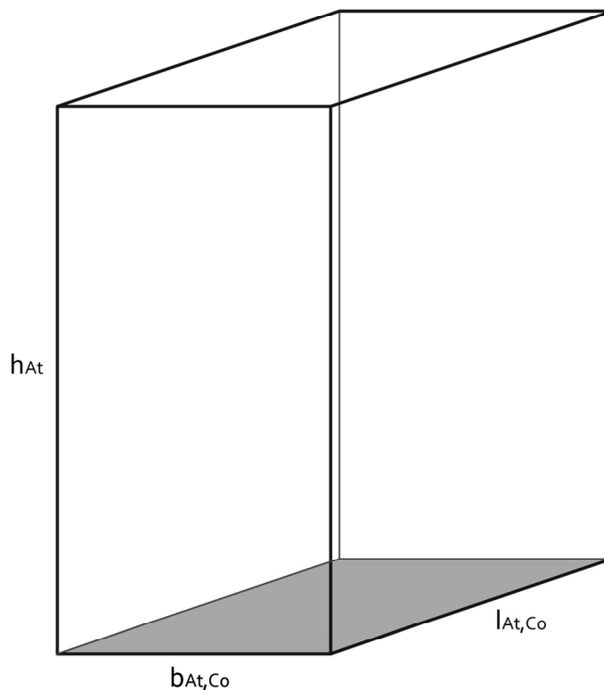
Figura 14 - Geometria di cortili ed atrii
